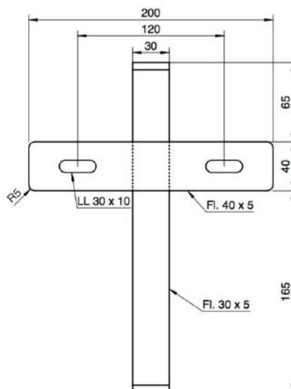
MASTHALTER VARIO-2
